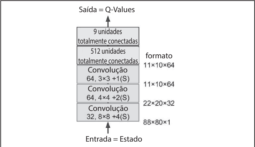
Figura 16-10. Q-network profunda para jogar Ms. Pac-Man
