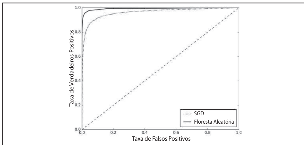
Figura 3-7. Comparando curvas ROC
