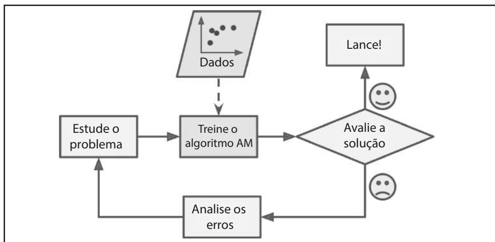
Figura 1-2. Abordagem do Aprendizado de Máquina
