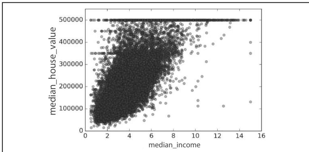
Figura 2-16. Renda média versus valor médio da habitação
