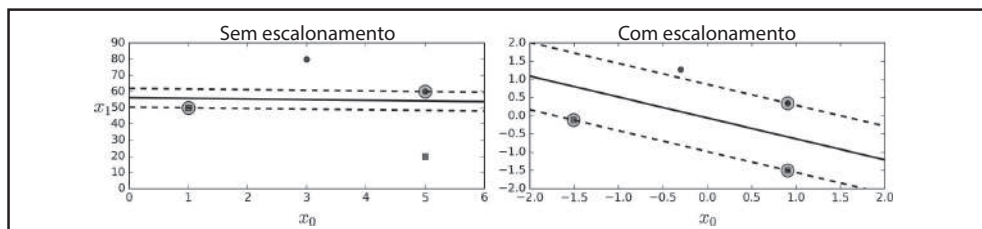
Figura 5-2. Sensitividade ao escalonamento das características
