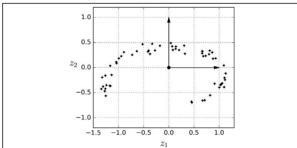
Figura 8-3. O novo conjunto de dados 2D após a projeção
