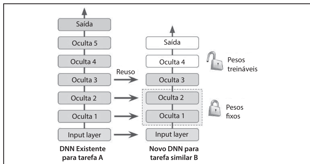
Figura 11-4. Reutilizando camadas pré-treinadas
