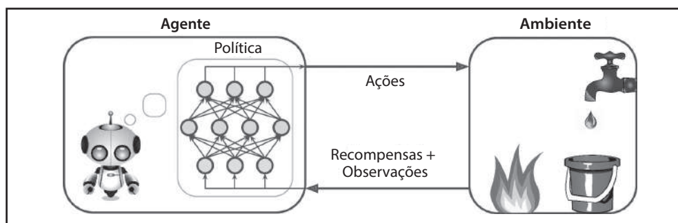
Figura 16-2. Aprendizado por reforço utilizando uma política de rede neural
