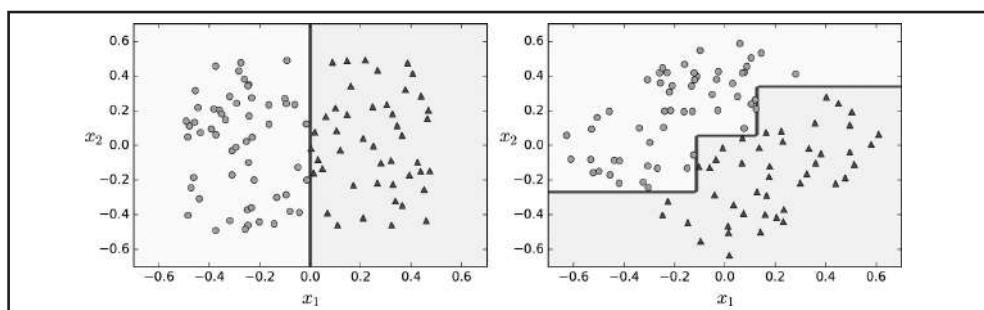
Figura 6-7. Sensibilidade à rotação no conjunto de treinamento
