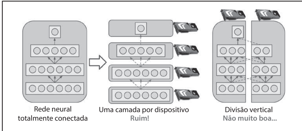
Figura 12-14. Divisão de uma rede neural totalmente conectada
