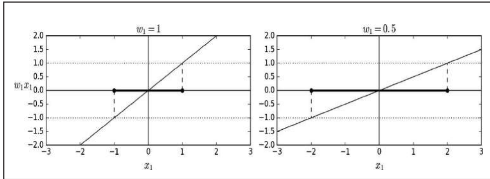
Figura 5-13. Um vetor de peso menor resulta em uma margem maior
