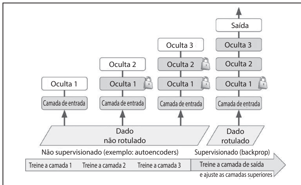
Figura 11-5. Pré-treinamento sem supervisão
