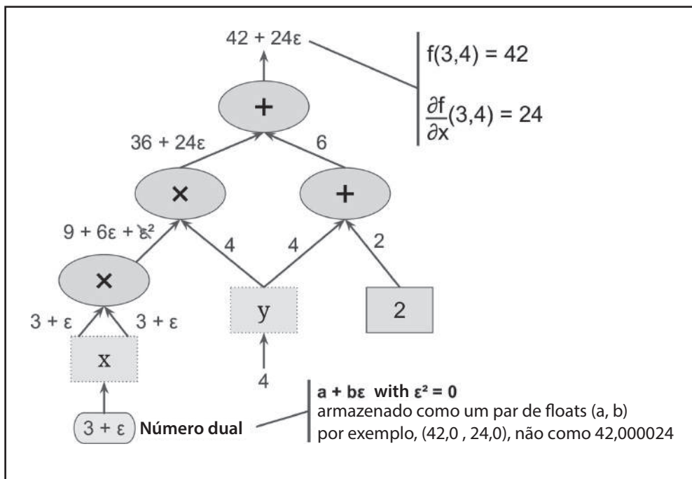
Figura D-2. Autodiff no Modo Forward
