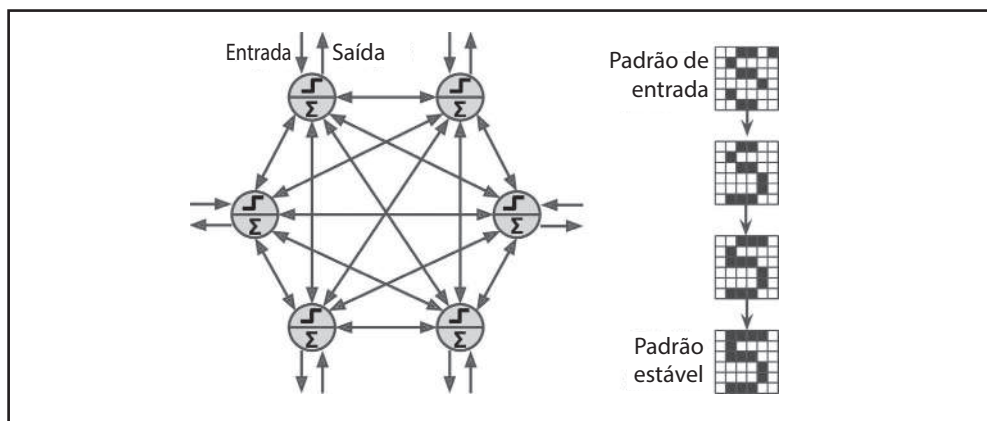
Figura E-1. Rede Hopfield
