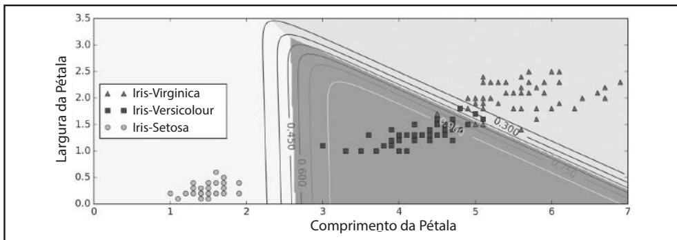
Figura 4-25. As fronteiras de decisão da Regressão Softmax
