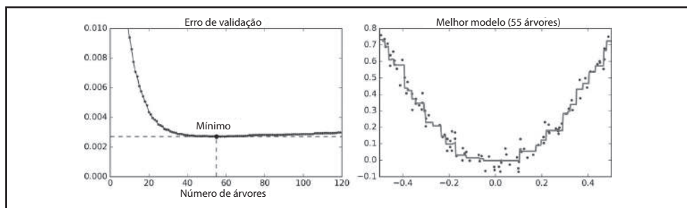
Figura 7-11. Ajustando o número de árvores utilizando uma parada antecipada
