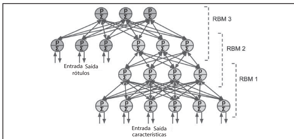
Figura E-4. Uma rede de crença profunda configurada para aprendizado semissupervisionado
