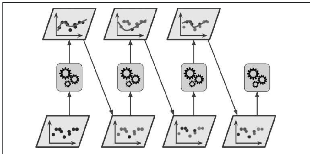
Figura 7-7. Treinamento sequencial AdaBoost com atualizações de peso das instâncias
