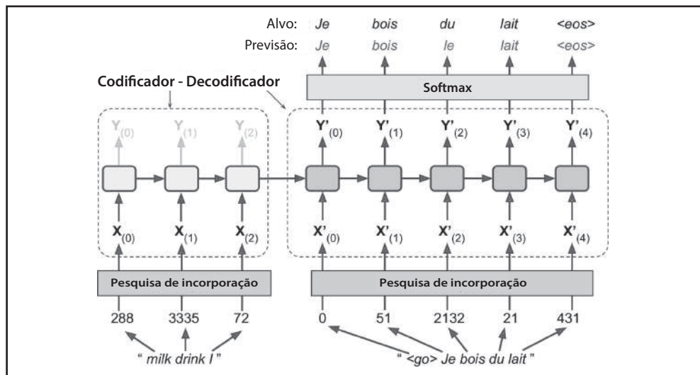
Figura 14-15. Um modelo simples de máquina de tradução
