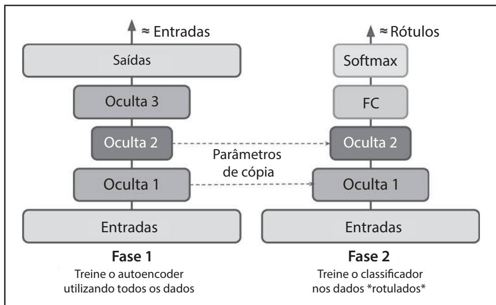
Figura 15-8. Pré-treinamento não supervisionado utilizando autoencoders
