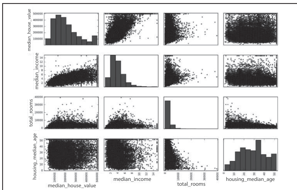
Figura 2-15. Matriz de dispersão
