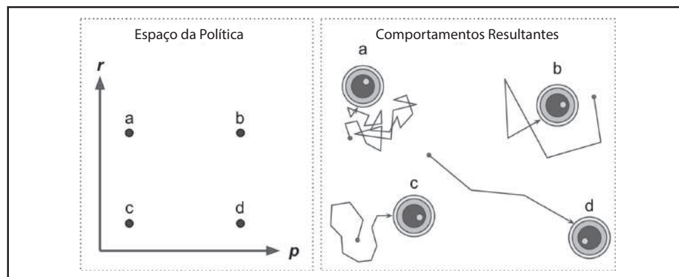
Figura 16-3. Quatro pontos no espaço da política e o comportamento correspondente do agente
