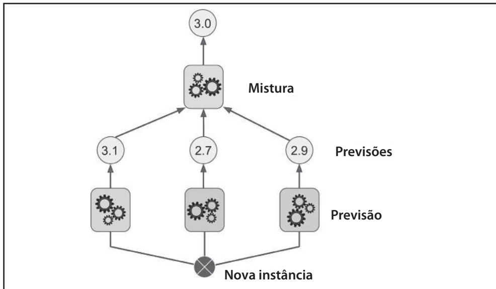
Figura 7-12. Agregando previsões com um predictor blender
