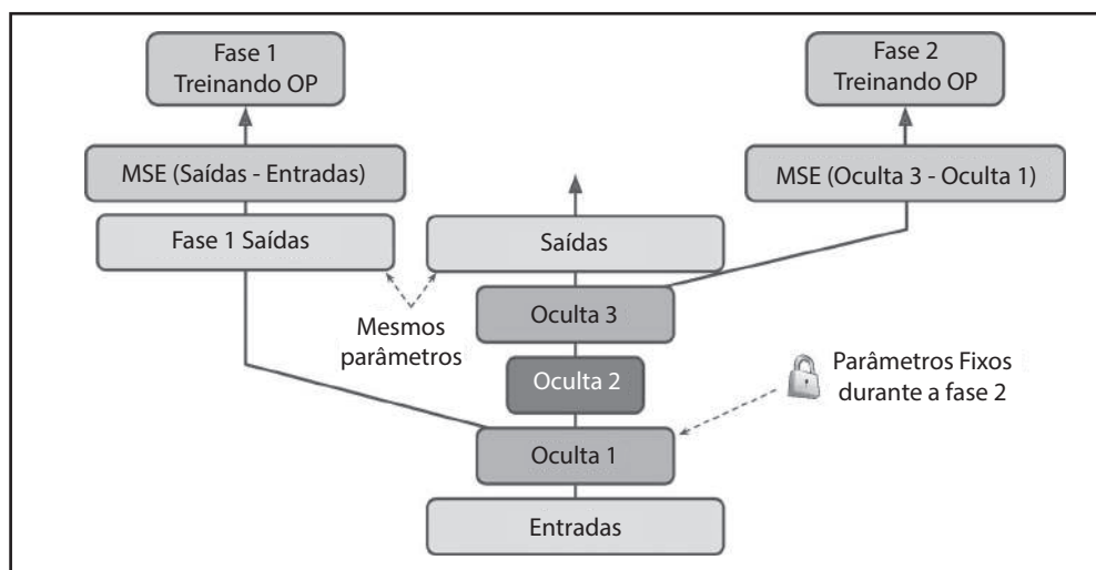
Figura 15-5. Um único grafo para treinar um autoencoder empilhado
