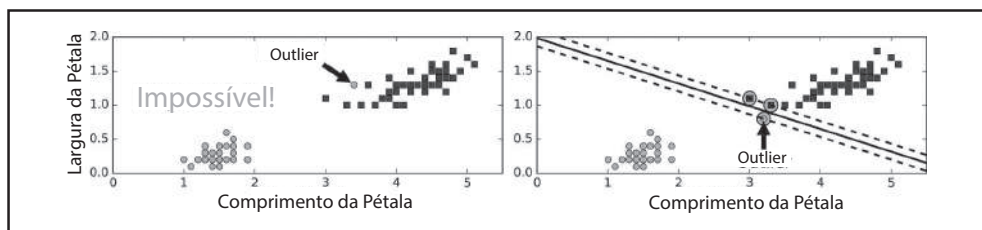
Figura 5-3. Sensibilidade da margem rígida aos outliers
