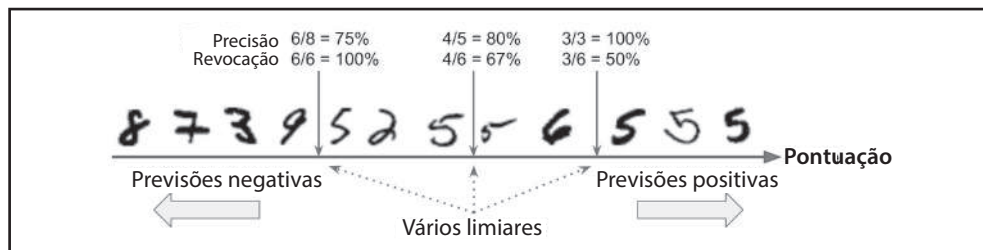
Figura 3-3. Limiar de decisão e compensação de precisão/revocação
