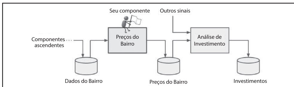
Figura 2-2. Um pipeline de Aprendizado de Máquina para investimentos imobiliários
