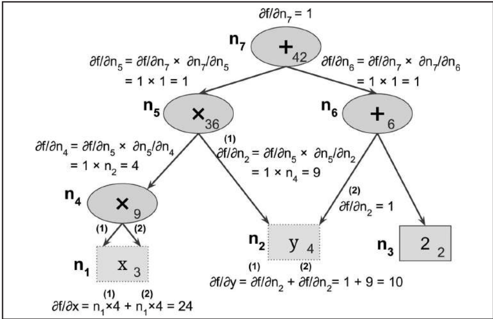
Figura D-3. Autodiff no Modo Reverso
