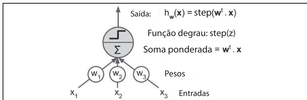
Figura 10-4. Unidade Linear com Threshold
