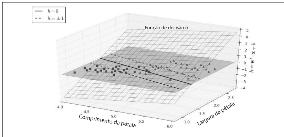
Figura 5-12. Função de decisão para o conjunto de dados da íris
