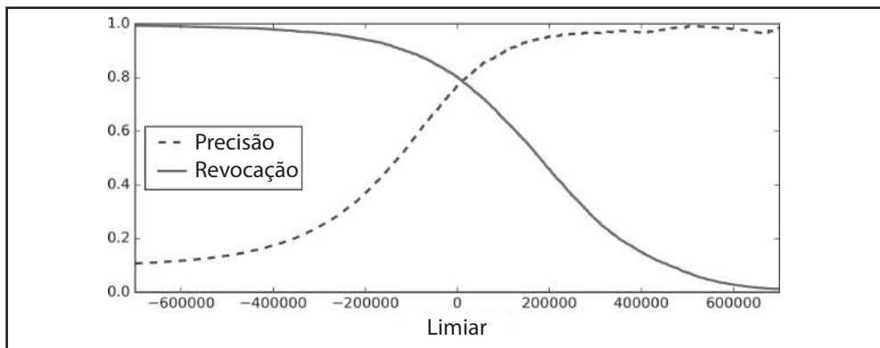
Figura 3-4. Precisão e revocação versus o limiar de decisão
