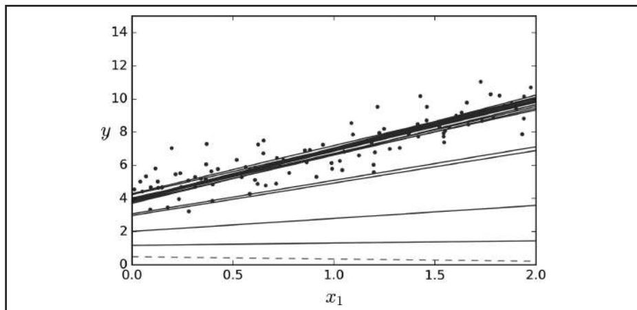
Figura 4-10. Os primeiros 10 passos do Gradiente Descendente Estocástico
