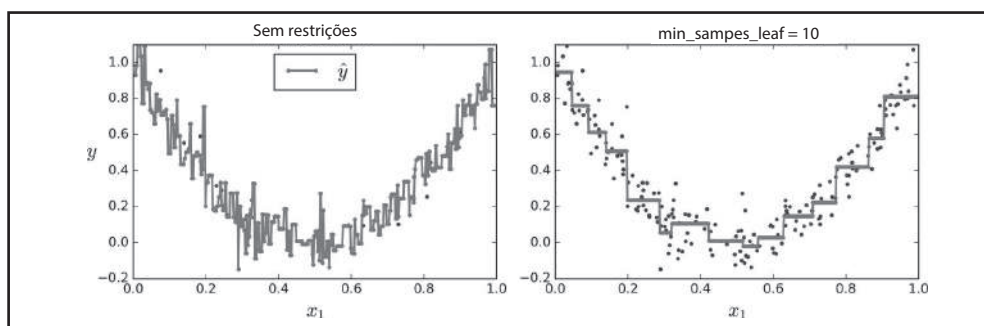
Figura 6-6. Regularizando um regressor da Árvore de Decisão
