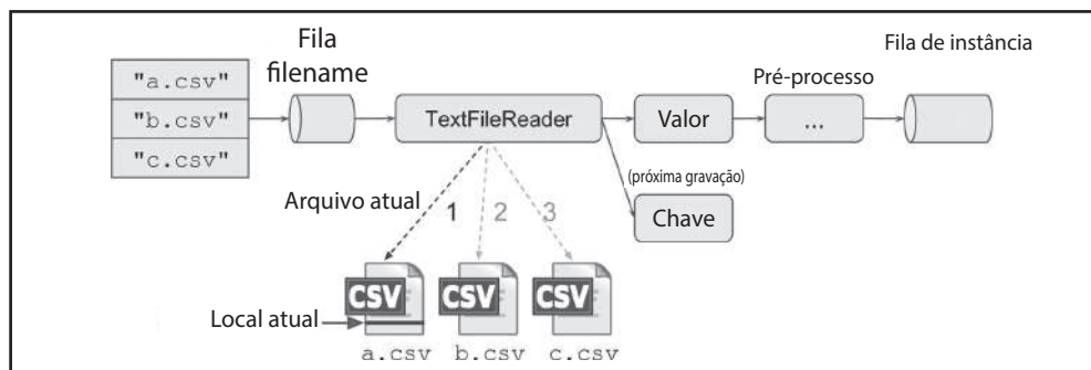
Figura 12-9. Um grafo dedicado à leitura de instâncias de treinamento de arquivos CSV
