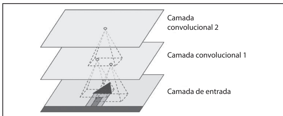
Figura 13-2. Camadas CNN com campos receptivos locais retangulares
