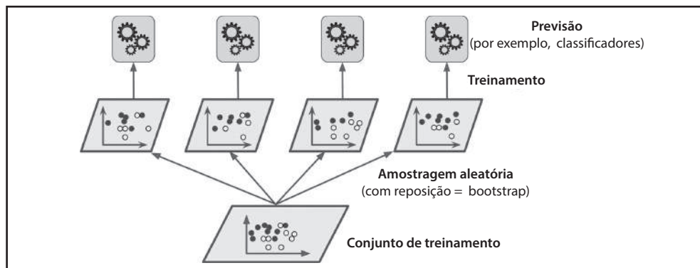
Figura 7-4. Conjunto de treinamento e amostragem pasting/bagging
