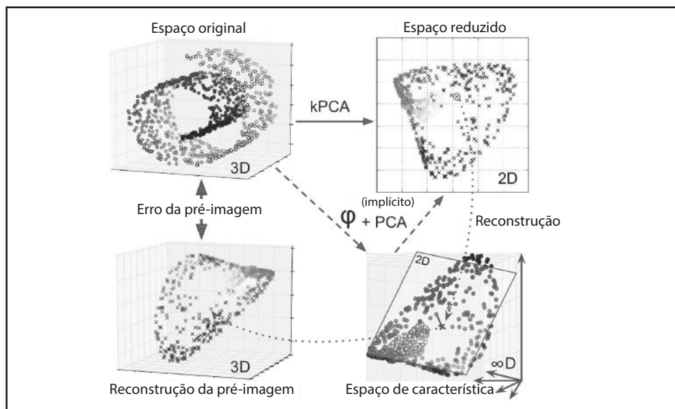
Figura 8-11. Kernel PCA e o erro de reconstrução da pré-imagem
