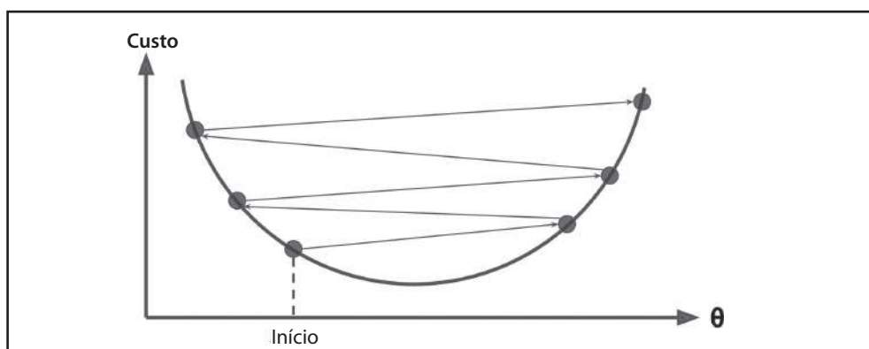
Figura 4-5. Taxa de aprendizado muito grande
