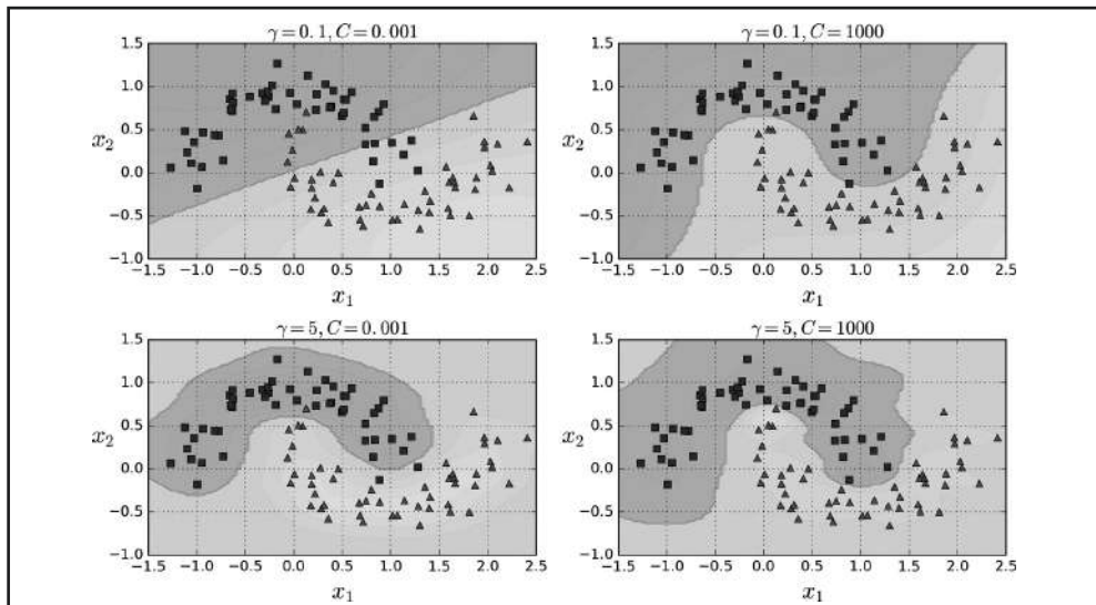
Figura 5-9. Classificadores SVM utilizando o kernel RBF
