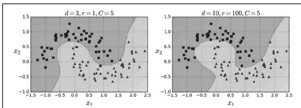
Figura 5-7. Classificadores SVM com um kernel polinomial
