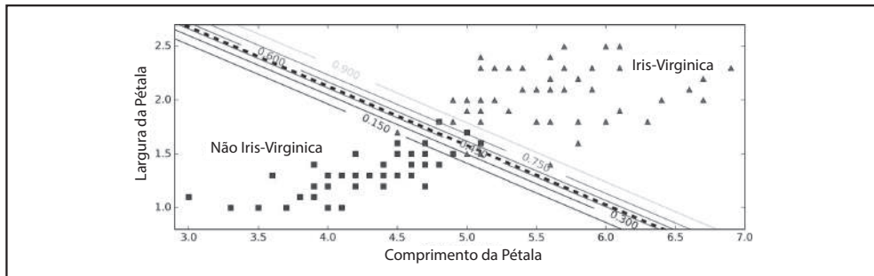
Figura 4-24. Fronteiras de decisão linear
