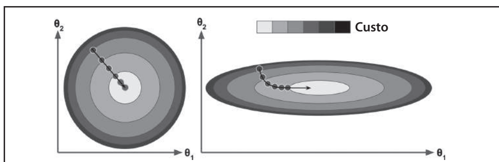
Figura 4-7. Gradiente Descendente com e sem escalonamento das características
