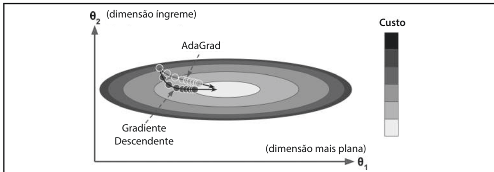
Figura 11-7. AdaGrad versus Gradiente Descendente
