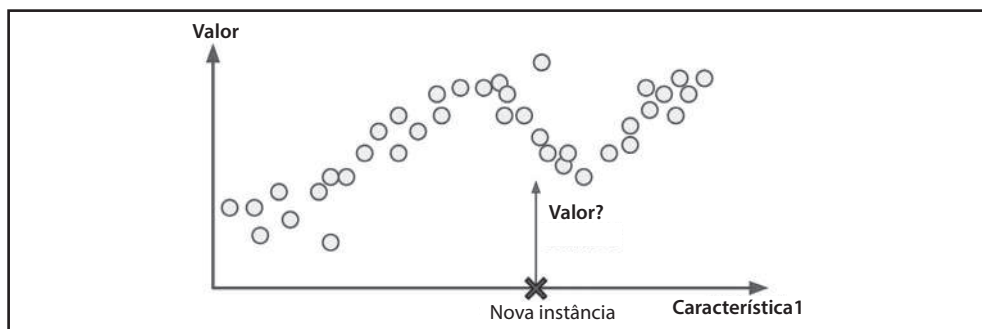
Figura 1-6. Regressão
