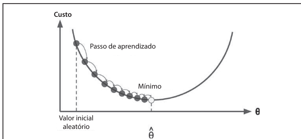
Figura 4-3. Gradiente Descendente
