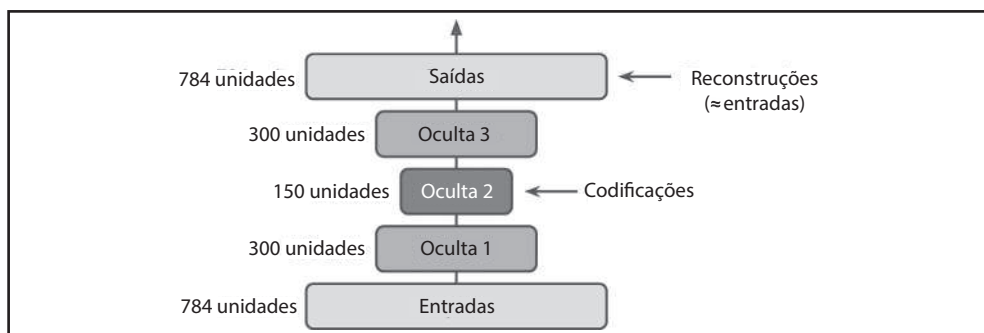
Figura 15-3. Autoencoder Empilhado
