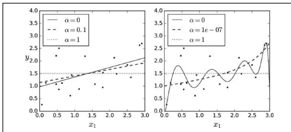
Figura 4-18. Regressão Lasso
