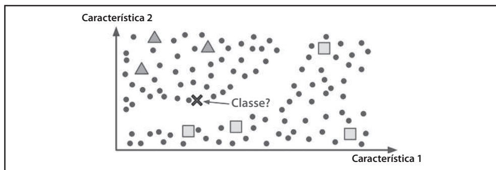
Figura 1-11. Aprendizado Semissupervisionado
