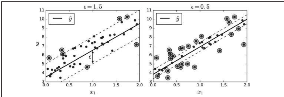
Figura 5-10. Regressão SVM
