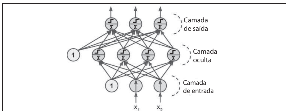
Figura 10-7. Multicamada Perceptron
