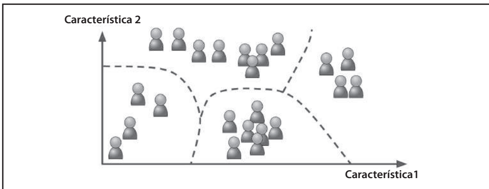
Figura 1-8. Clustering
