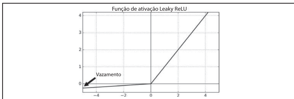
Figura 11-2. Leaky ReLU
