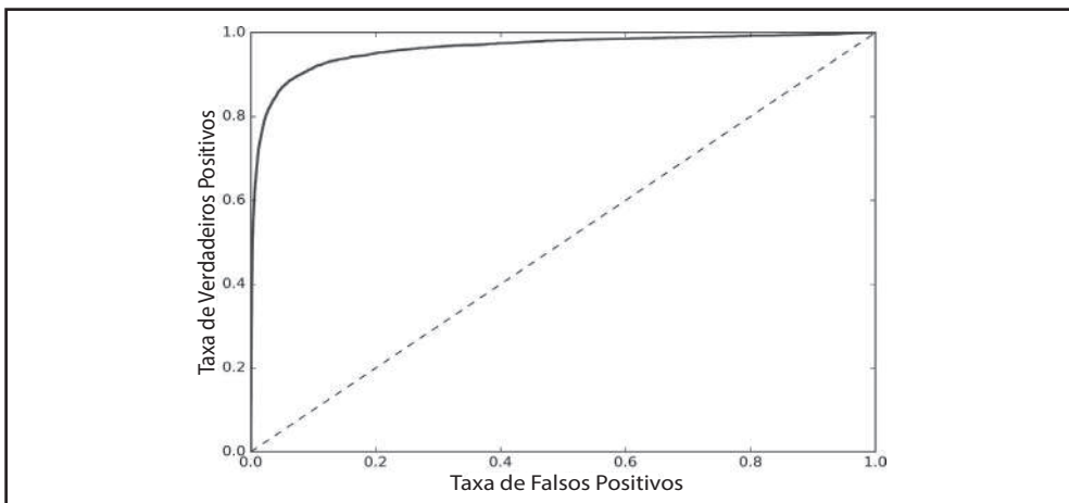
Figura 3-6. Curva ROC
