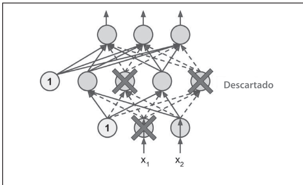
Figura 11-9. Regularização Dropout
