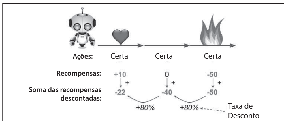
Figura 16-6. Recompensas descontadas
