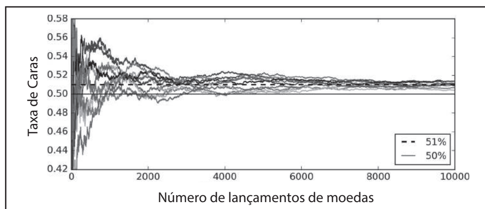
Figura 7-3. A lei dos grandes números
