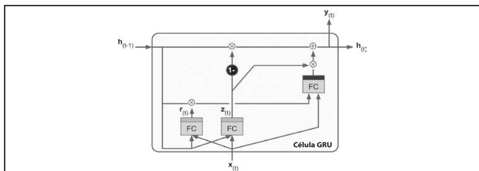
Figura 14-14. Célula GRU
