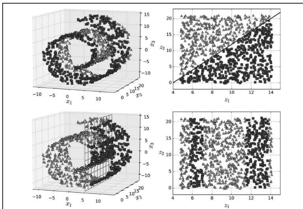
Figura 8-6. A fronteira de decisão nem sempre é mais simples com dimensões inferiores
