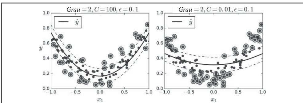
Figura 5-11. Regressão SVM utilizando um kernel polinomial de 2º grau
