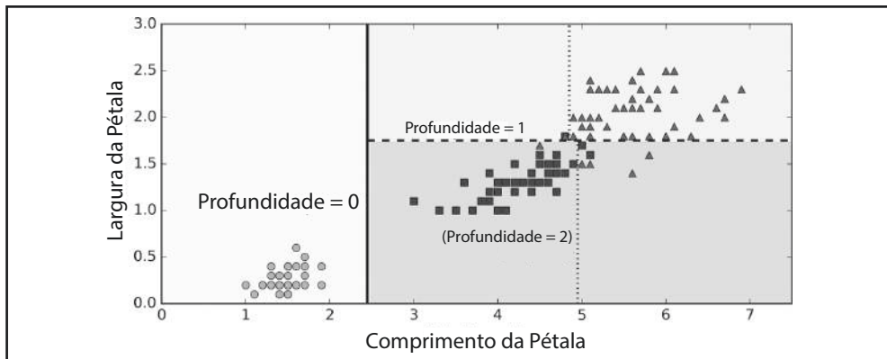
Figura 6-2. Fronteiras de decisão da Árvore de Decisão
