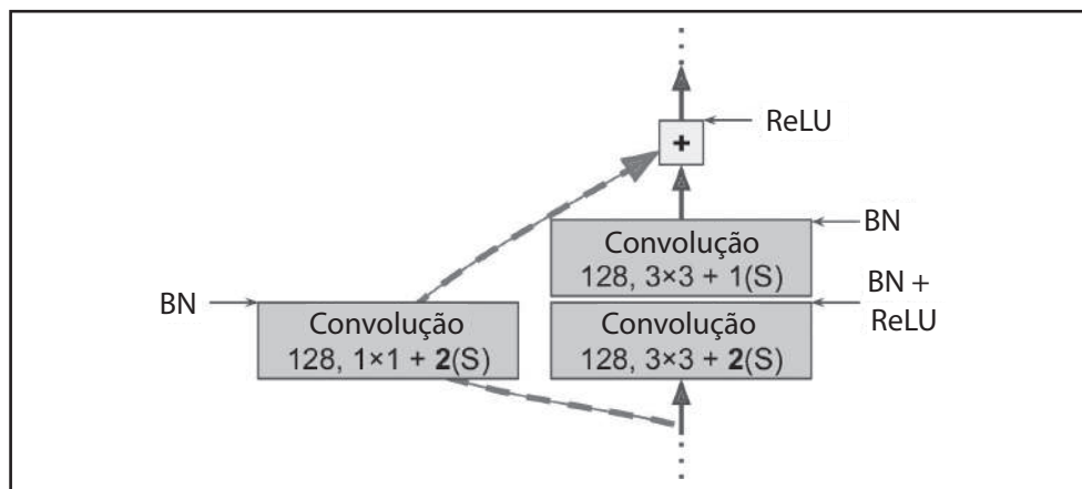
Figura 13-15. Conexão skip ao alterar o tamanho e a profundidade do mapa de características
