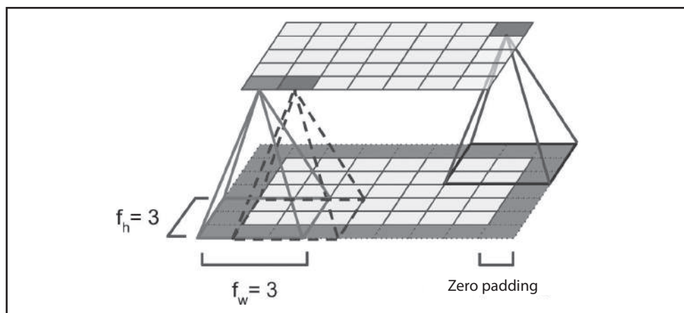
Figura 13-3. Conexões entre camadas e zero padding
