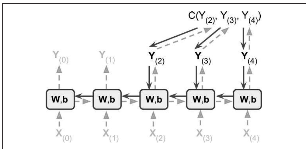
Figura 14-5. Retropropagação ao longo do tempo
