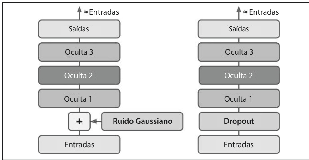
Figura 15-9. Autoencoders de Remoção de Ruído, com ruído Gaussiano (esquerda) ou dropout (direita)
