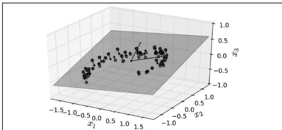
Figura 8-2. Um conjunto de dados 3D perto de um subespaço 2D
