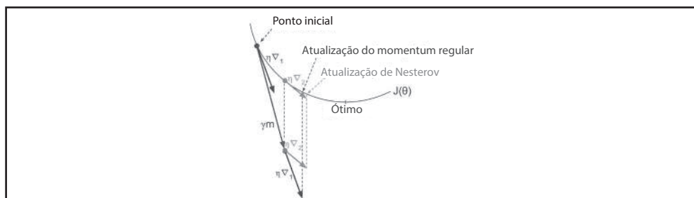
Figura 11-6. Otimização Regular versus otimização Momentum de Nesterov
