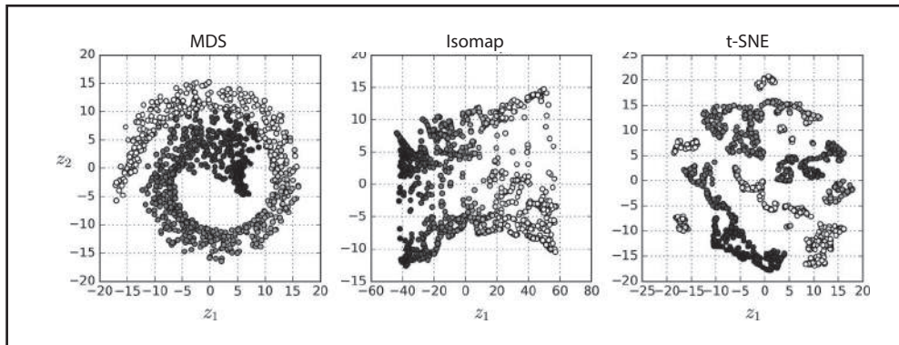
Figura 8-13. Reduzindo o rolo suíço para 2D com a utilização de várias técnicas
