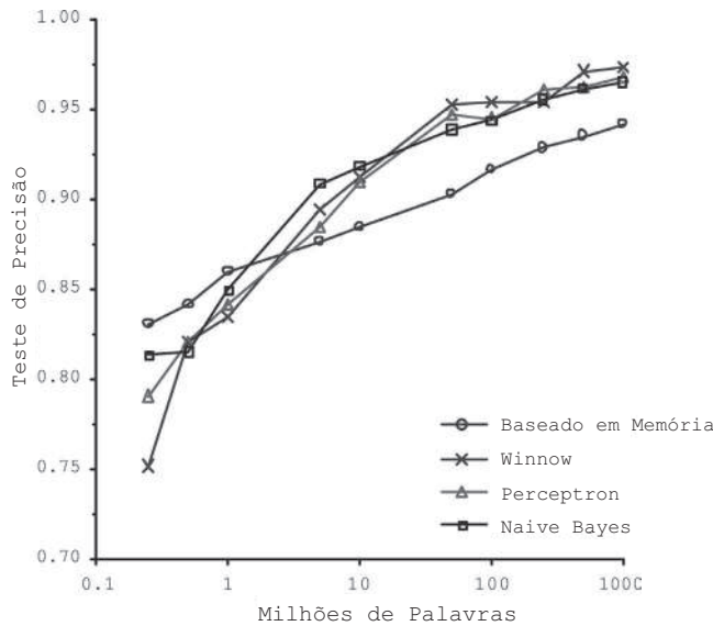
Figura 1-20. A importância dos dados versus algoritmos 9
