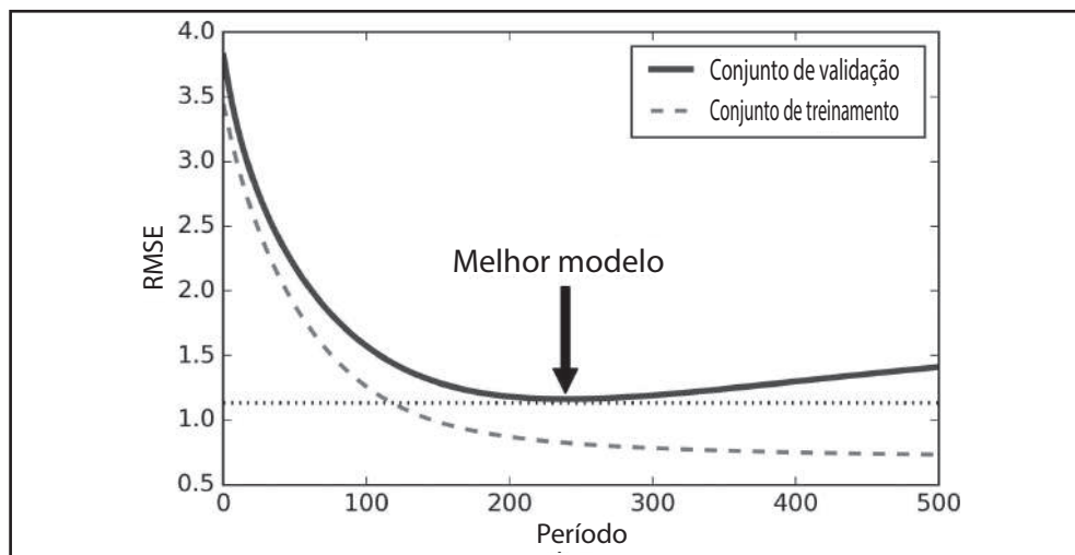
Figura 4-20. Regularização da Parada Antecipada
