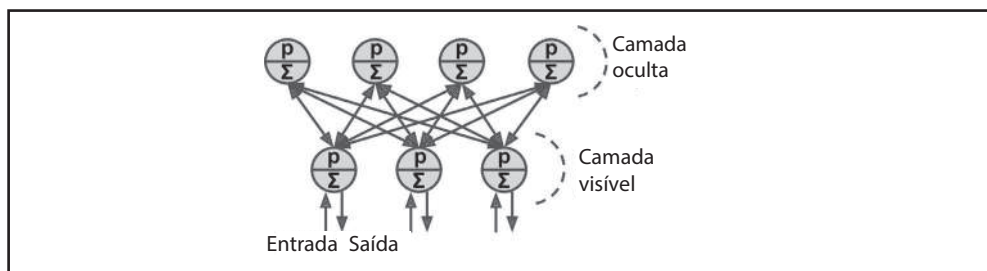
Figura E-3. Máquina Restrita de Boltzmann
