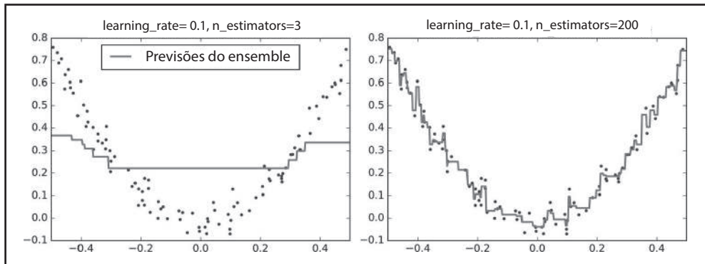
Figura 7-10. Ensembles GBRT com previsores insuficientes (à esquerda) e demais (à direita)
