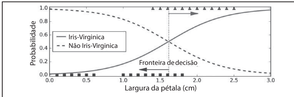
Figura 4-23. Probabilidades estimadas e limites da decisão
