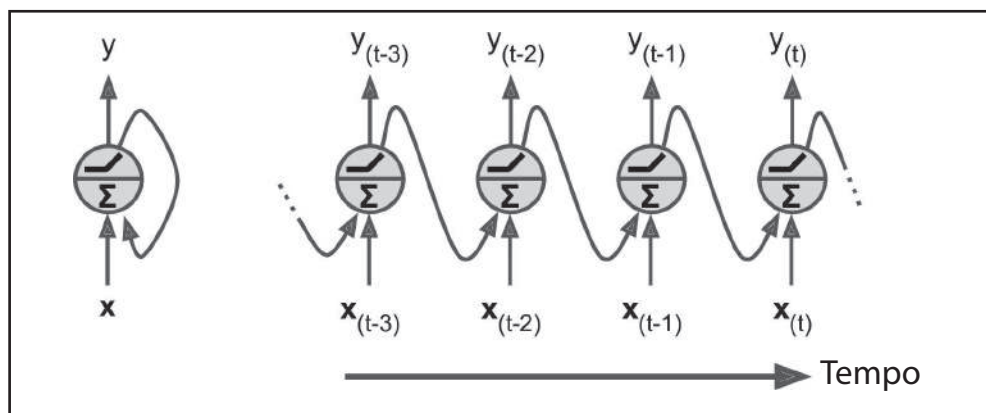
Figura 14-1. Um neurônio recorrente (esquerda), desenrolado através do tempo (direita)
