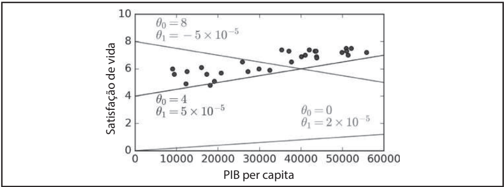
Figura 1-18. Alguns modelos lineares possíveis
