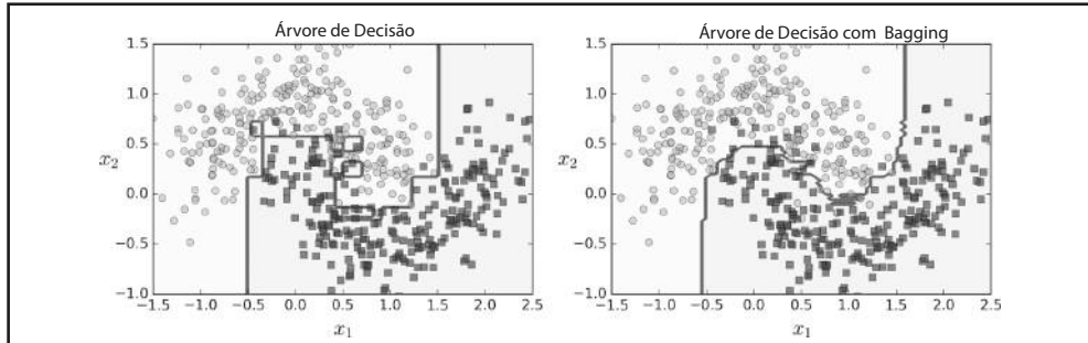
Figura 7-5. Uma Árvore de Decisão única versus um bagging ensemble de 500 árvores
