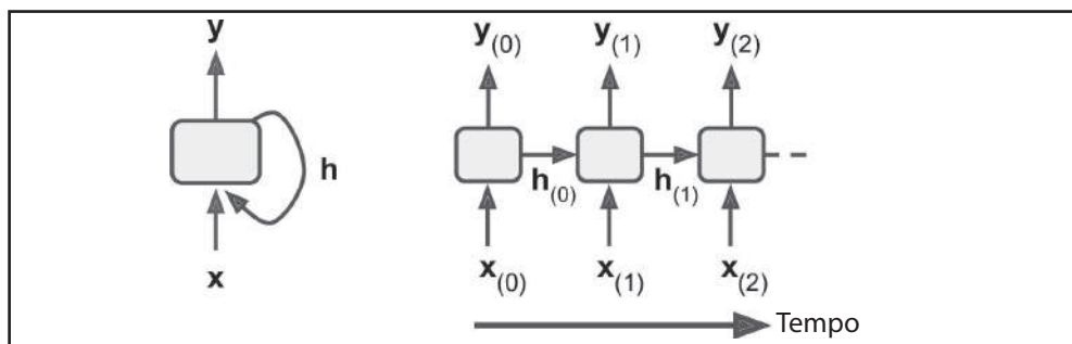
Figura 14-3. O estado oculto de uma célula e sua saída podem ser diferentes
