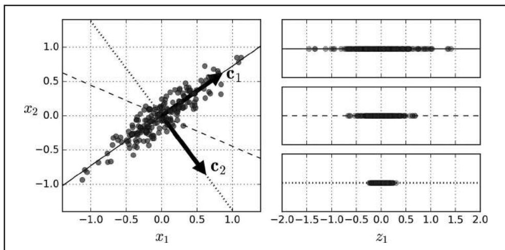
Figura 8-7. Selecionando o subespaço no qual projetar
