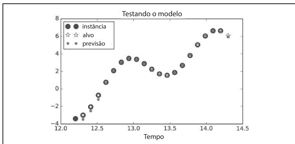
Figura 14-9. Previsões de séries temporais
