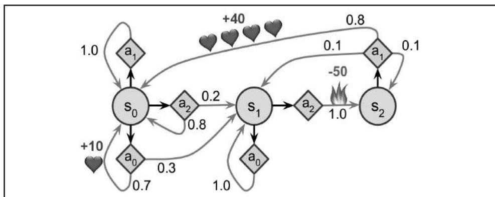
Figura 16-8. Exemplo de um processo de decisão de Markov
