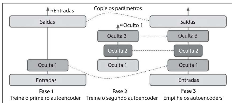
Figura 15-4. Treinando um autoencoder por vez
