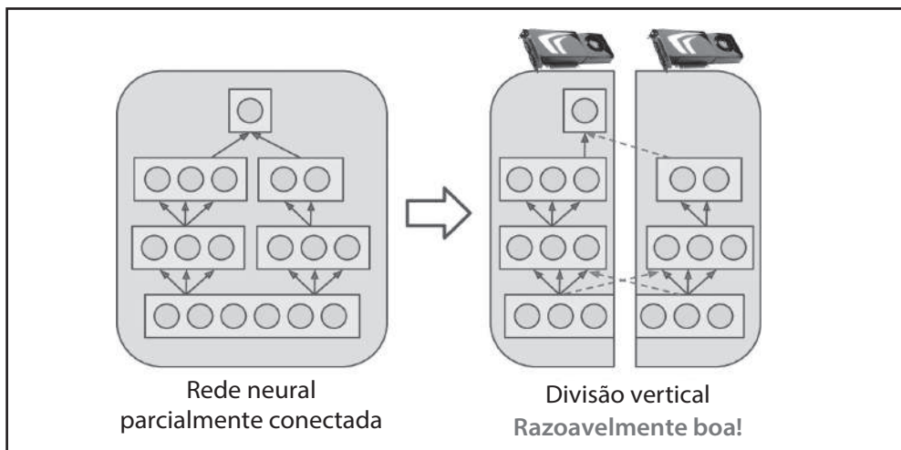
Figura 12-15. Dividindo uma rede neural parcialmente conectada
