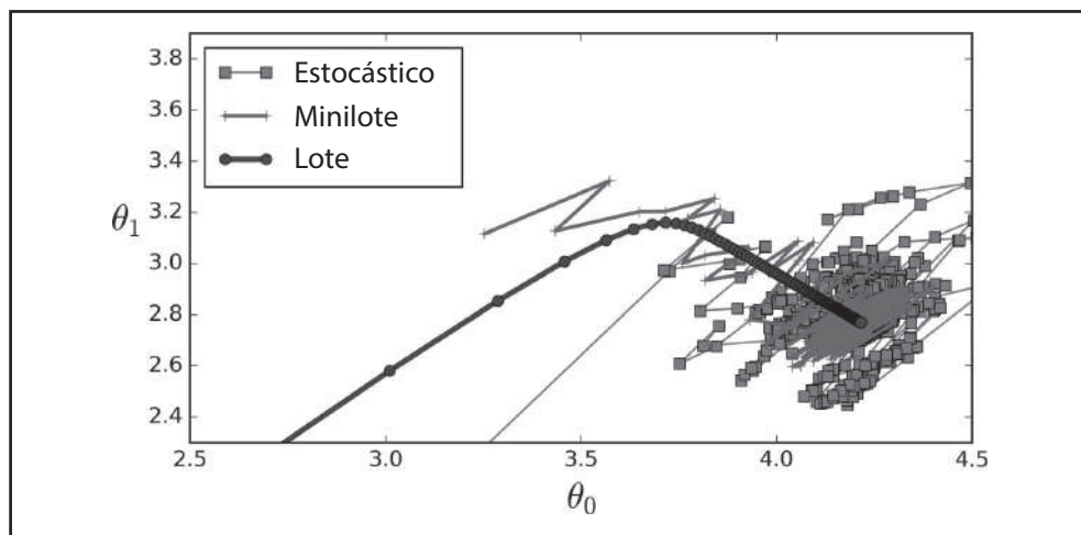
Figura 4-11. Caminhos do Gradiente Descendente no espaço de parâmetro
