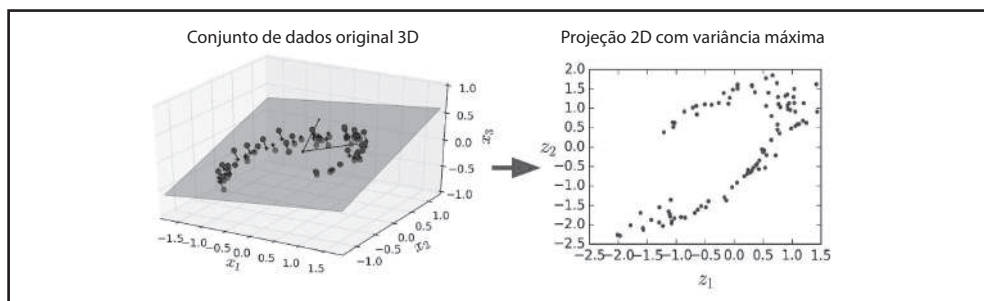
Figura 15-2. PCA realizada por um autoencoder linear incompleto
