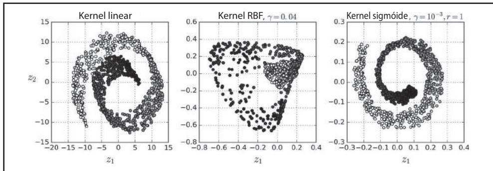
Figura 8-10. Rolo suíço reduzido para 2D utilizando kPCA com vários kernels
