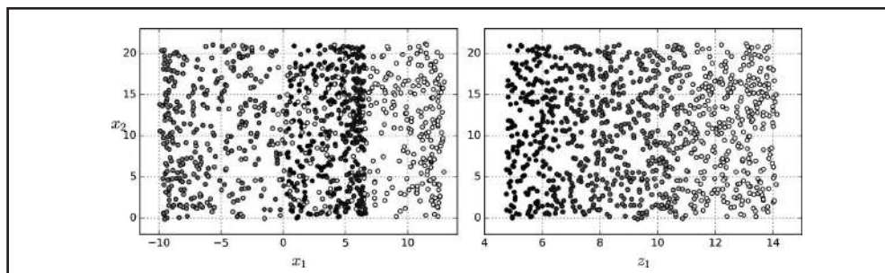
Figura 8-5. Esmagar o rolo ao projetá-lo em um plano (esquerda) versus desenrolar o rolo suíço (direita)
