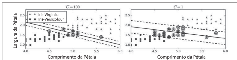
Figura 5-4. Menos violações de margem versus grandes margens
