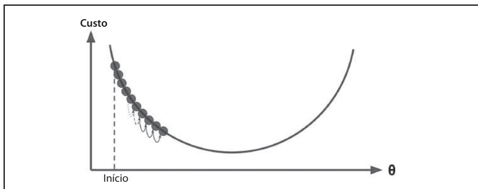
Figura 4-4. Taxa de aprendizado muito pequena
