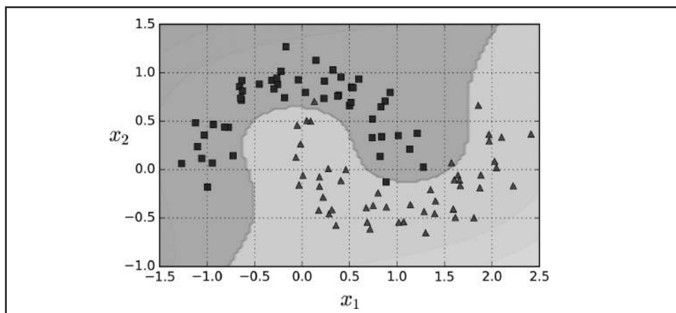
Figura 5-6. Classificador Linear SVM com a utilização de características polinomiais
