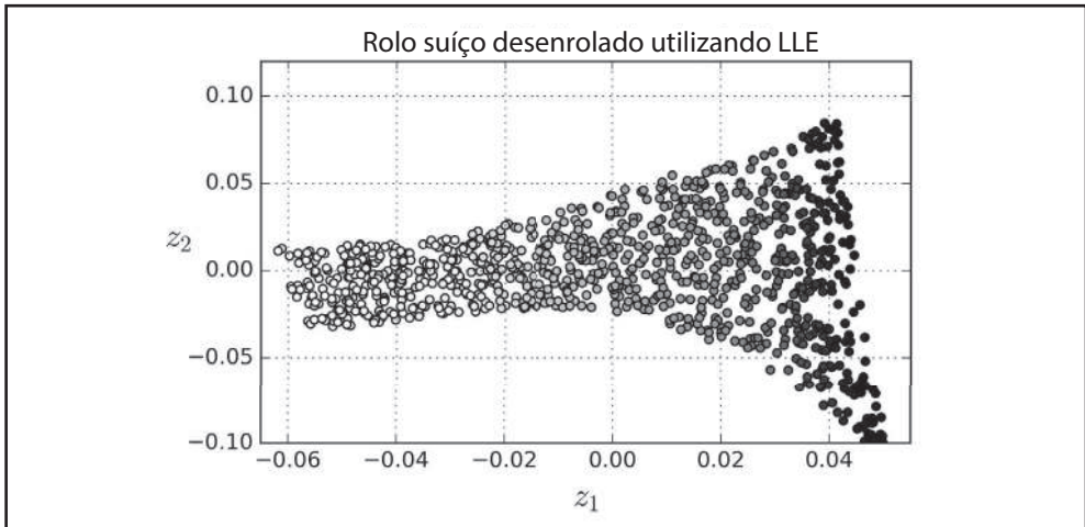
Figura 8-12. Rolo suíço desenrolado com a utilização do LLE
