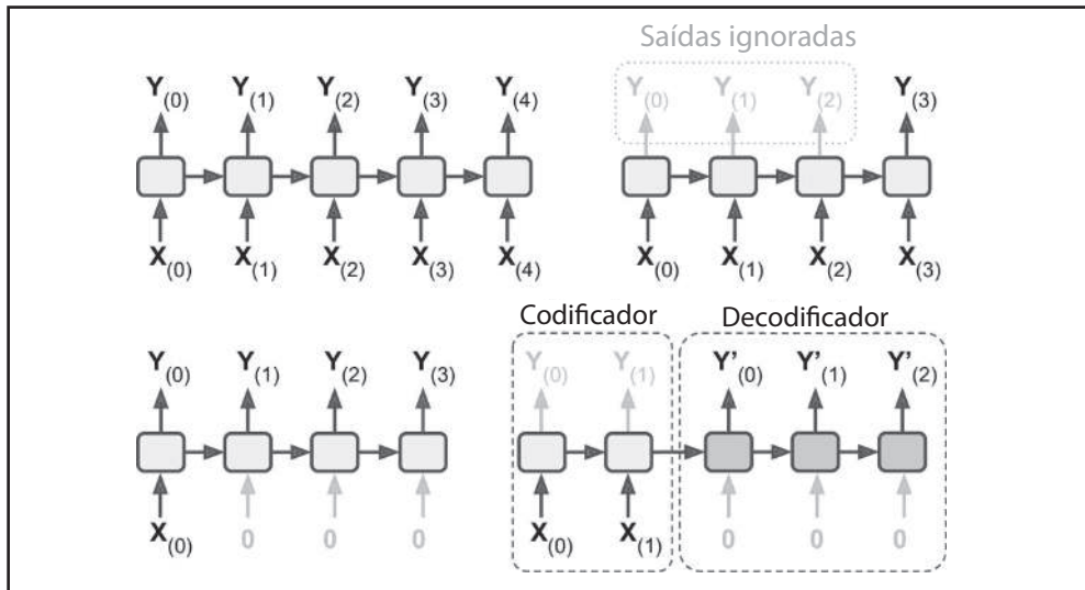
Figura 14-4. Seq para seq (canto superior esquerdo), seq para vetor (canto superior direito), vetor para seq (canto inferior esquerdo), delayed seq para seq (canto inferior direito)
