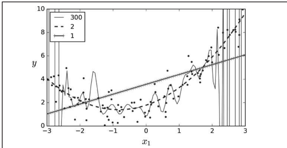
Figura 4-14. Regressão Polinomial de Grau Elevado
