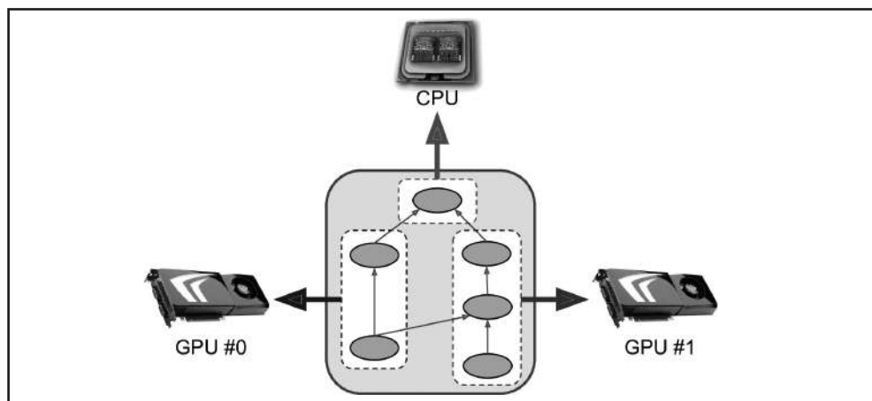
Figura 12-1. Executando um grafo do TensorFlow em múltiplos dispositivos paralelos
