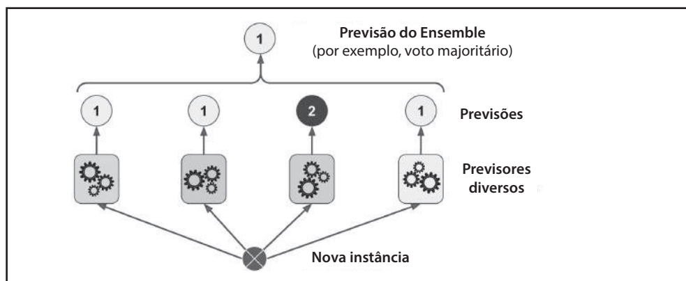
Figura 7-2. Previsões do classificador hard voting
