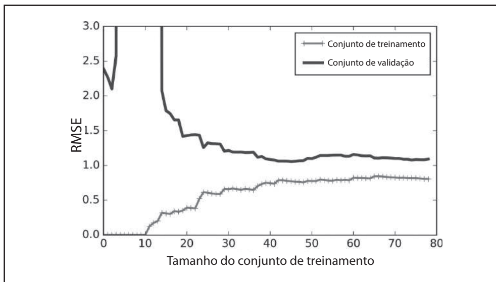
Figura 4-16. Curvas de Aprendizado para o modelo polinomial
