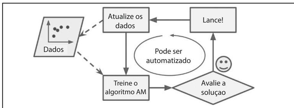
Figura 1-3. Adaptando-se automaticamente à mudança
