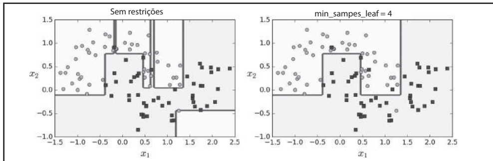
Figura 6-3. Regularização utilizando min_samples_leaf
