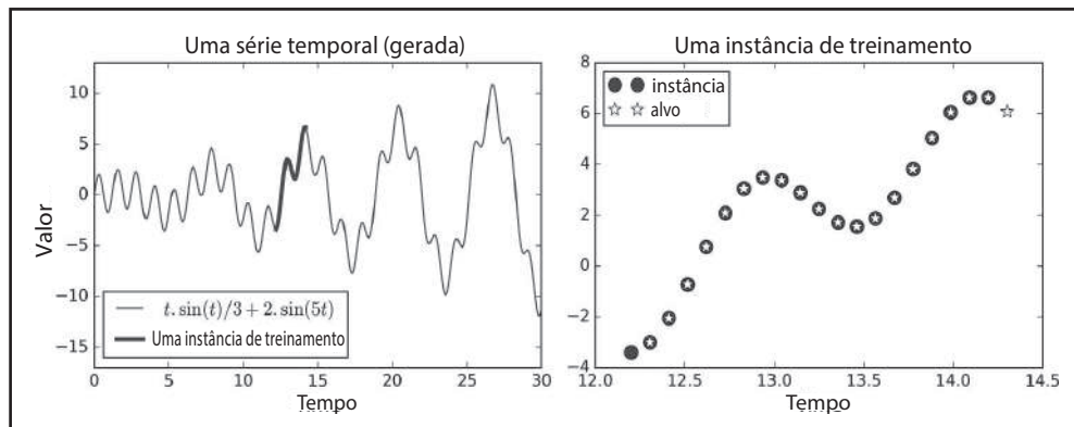
Figura 14-7. Séries temporais (à esquerda) e uma instância de treinamento dessa série (à direita)
