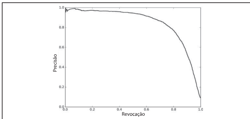
Figura 3-5. Precisão versus revocação
