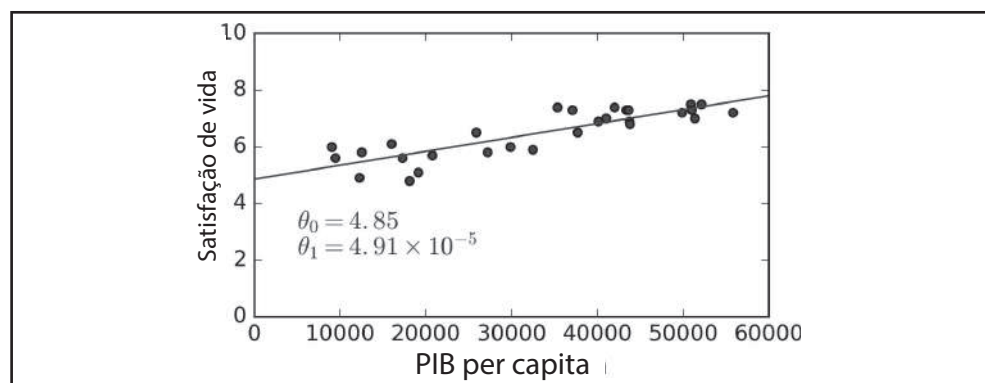
Figura 1-19. O modelo linear que melhor se ajusta aos dados de treinamento
