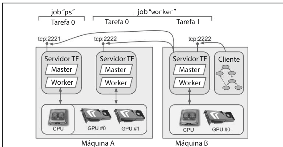
Figura 12-6. Cluster do TensorFlow
