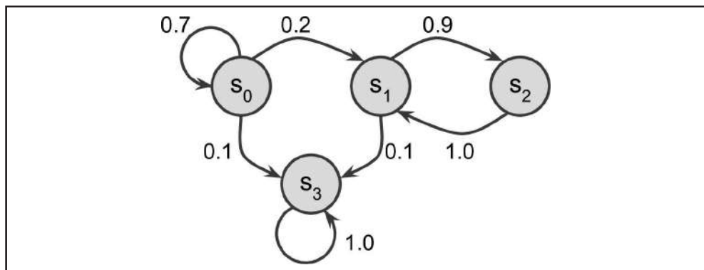
Figura 16-7. Exemplo de uma cadeia de Markov
