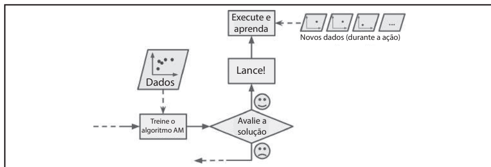
Figura 1-13. Aprendizado online
