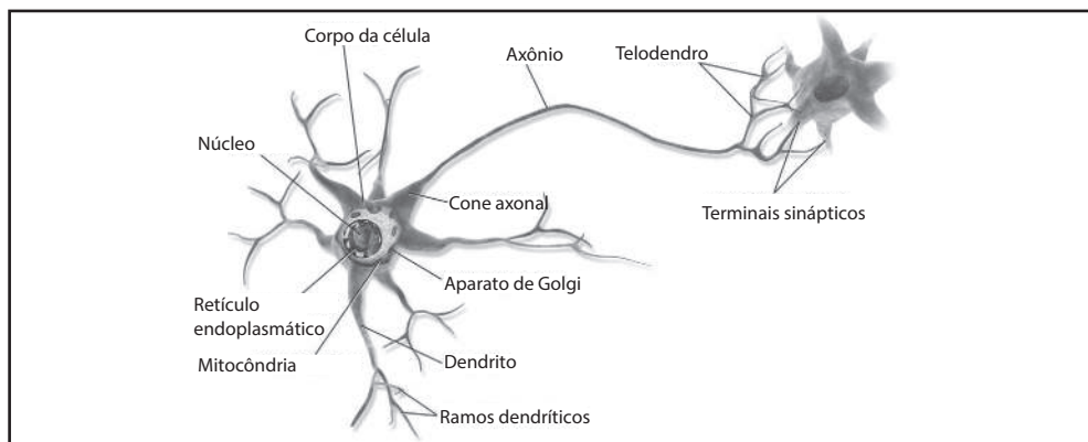
Figura 10-1. Neurônio Biológico 3
