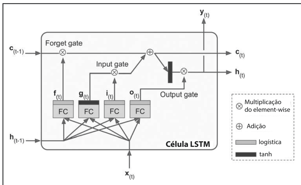
Figura 14-13. Célula LSTM
