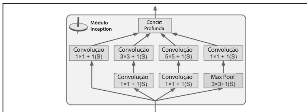
Figura 13-10. Módulo Inception
