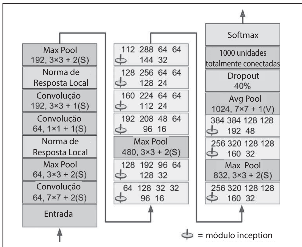
Figura 13-11. Arquitetura GoogLeNet
