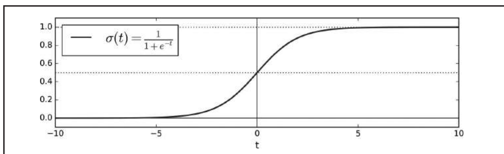
Figura 4-21. Função Logística
