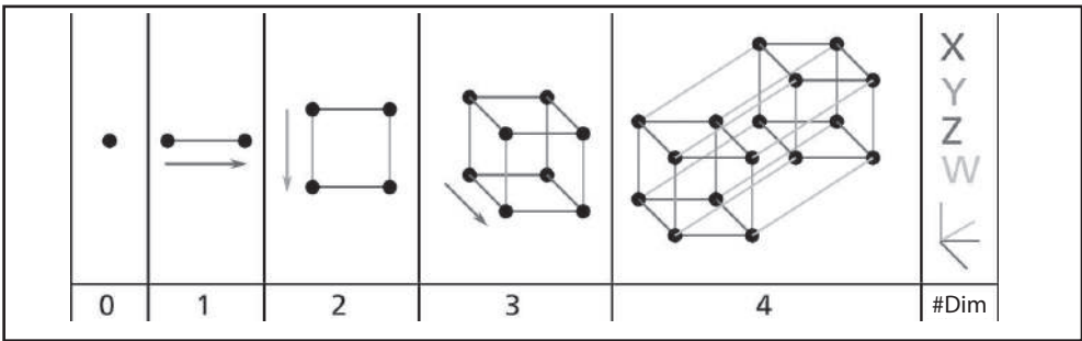
Figura 8-1. Ponto, segmento, quadrado, cubo e tesseracto (hipercubos 0D a 4D) 2
