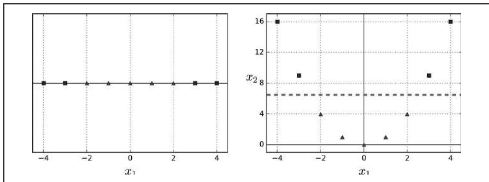
Figura 5-5. Adicionando características para tornar um conjunto de dados linearmente separável
