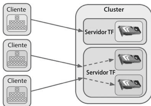
Figura 12-11. Treinando uma rede neural por dispositivo
