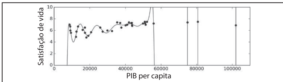
Figura 1-22. Sobreajustando nos dados de treinamento
