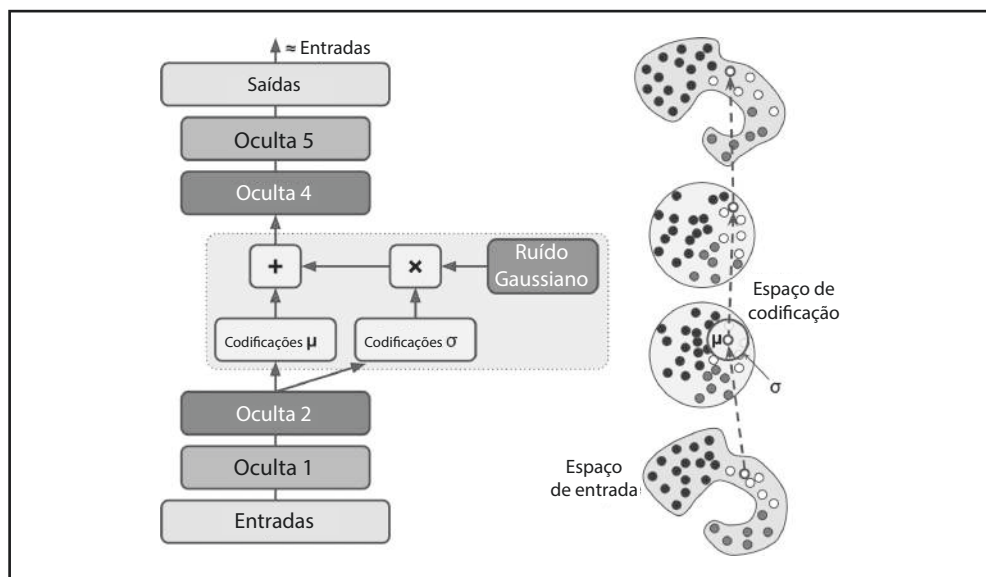
Figura 15-11. Autoencoder Variacional (esquerda) e uma instância passando por ele (direita)
