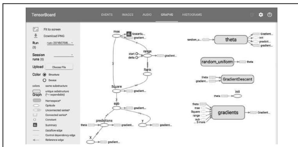
Figura 9-4. Visualizando o grafo com a utilização do TensorBoard
