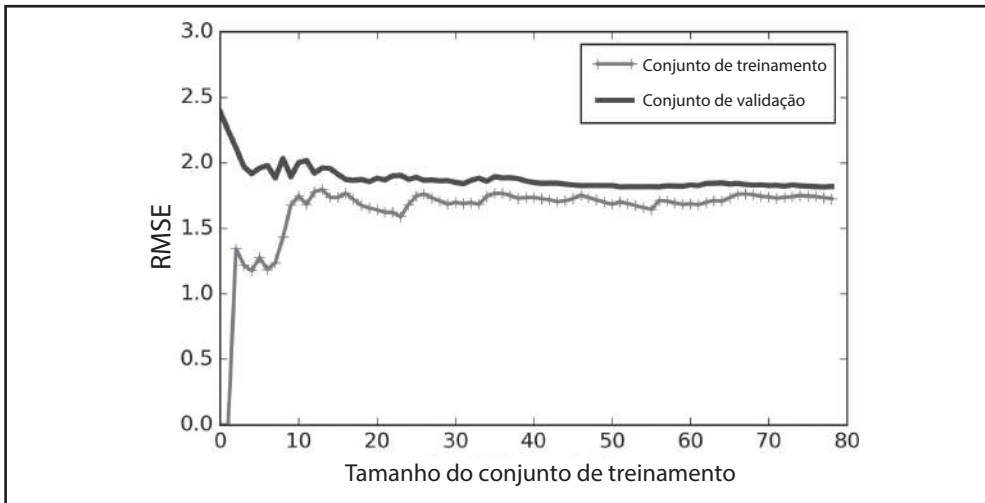
Figura 4-15. Curvas de Aprendizado
