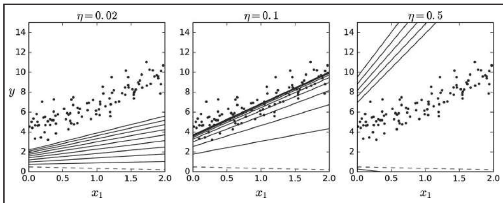
Figura 4-8. O Gradiente Descendente com várias taxas de aprendizado
