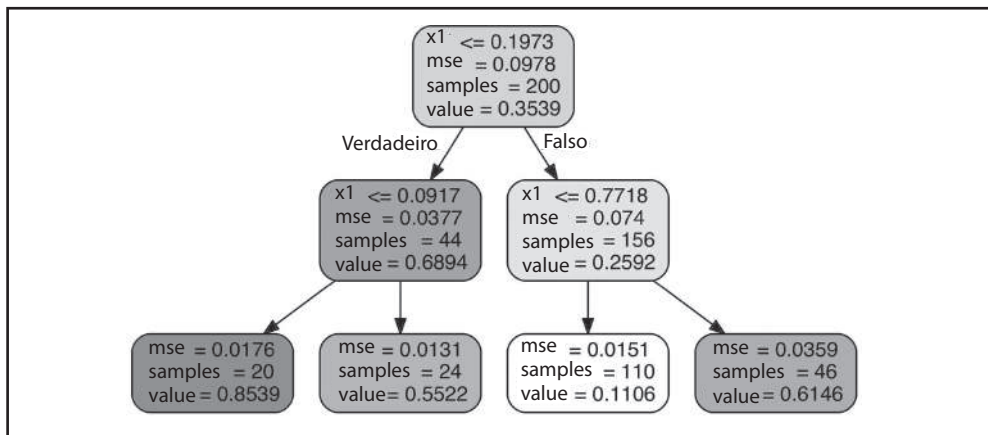
Figura 6-4. Uma Árvore de Decisão para regressão
