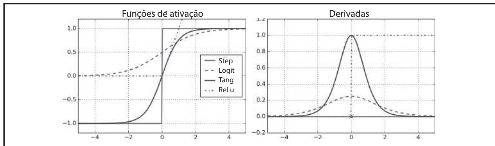
Figura 10-8. Funções de Ativação e suas derivadas
