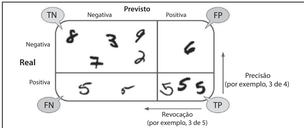
Figura 3-2. Uma matriz de confusão ilustrada
