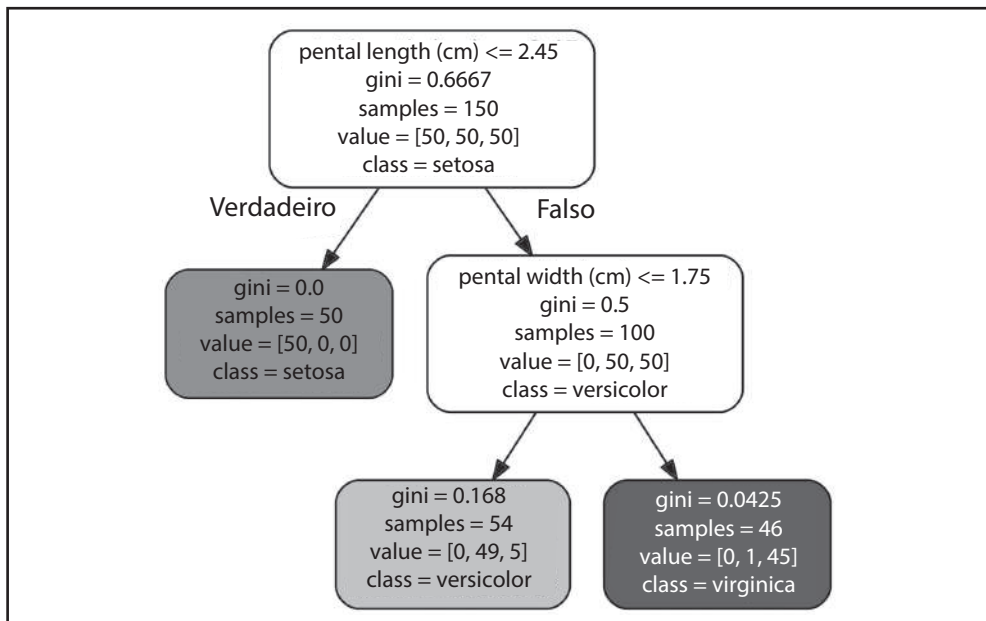
Figura 6-1. Árvore de Decisão da iris
