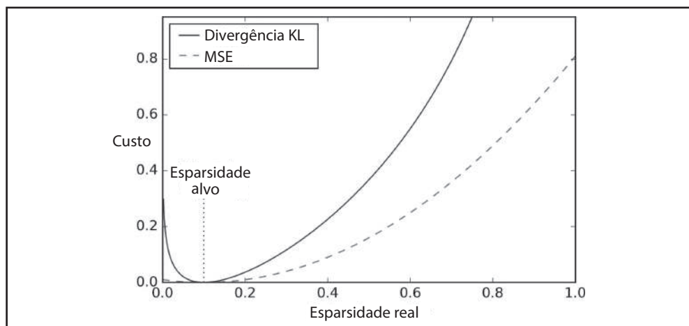
Figura 15-10. Perda de esparsidade
