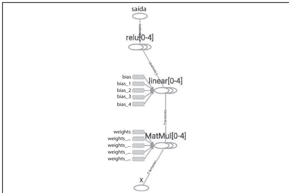
Figura 9-6. Séries de nós colapsados
