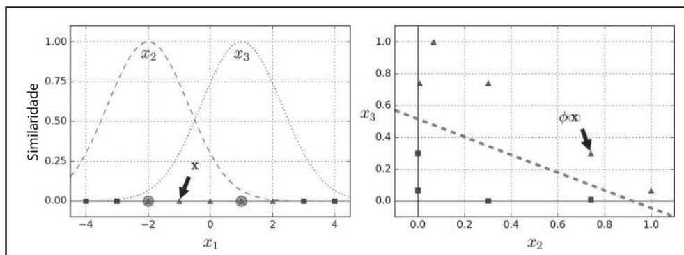
Figura 5-8. Características de similaridade utilizando a RBF Gaussiana
