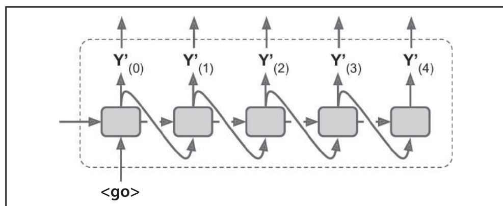
Figura 14-16. Alimentando a palavra de saída anterior como entrada no tempo de inferência
