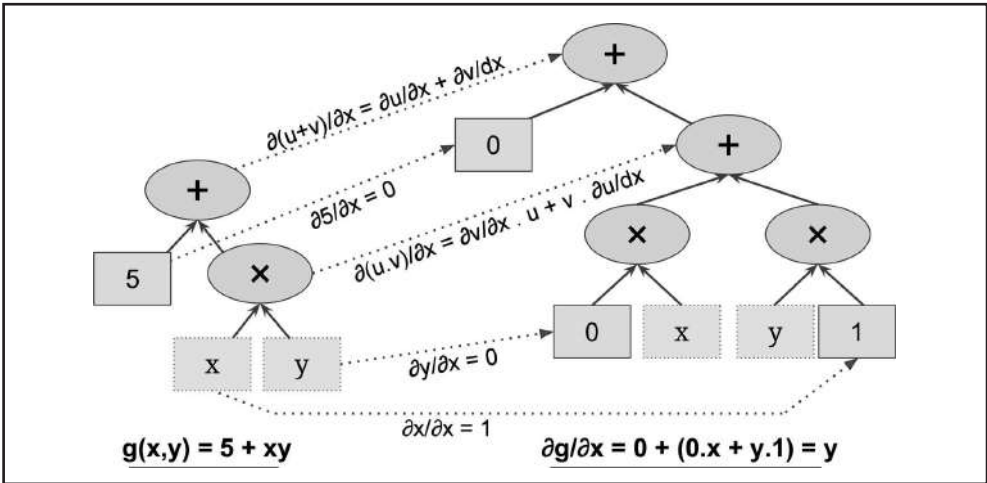
Figura D-1. Diferenciação Simbólica
