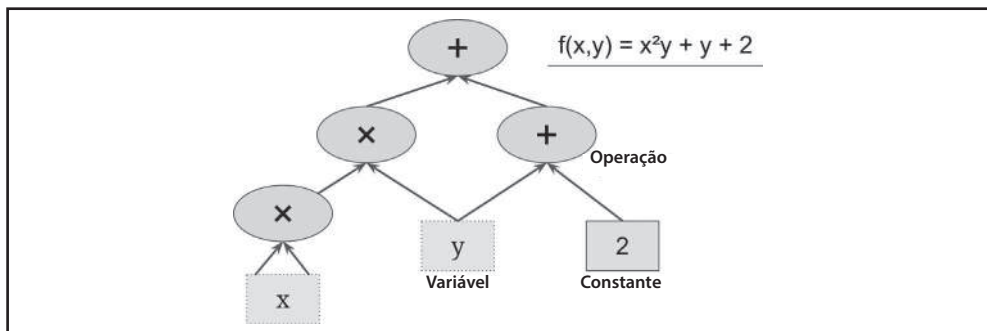
Figura 9-1. Um grafo de cálculo simples
