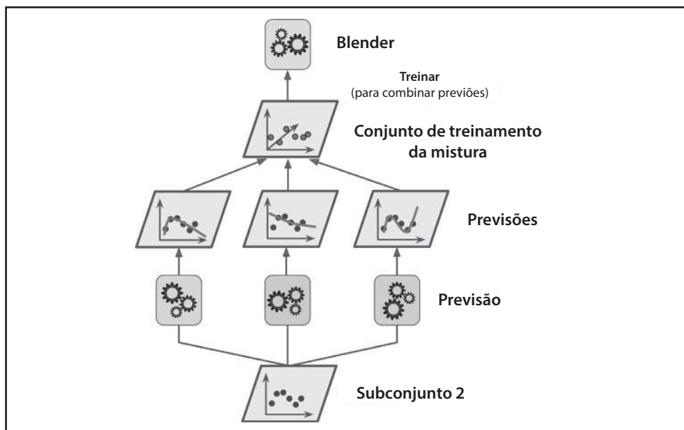
Figura 7-14. Treinando o blender
