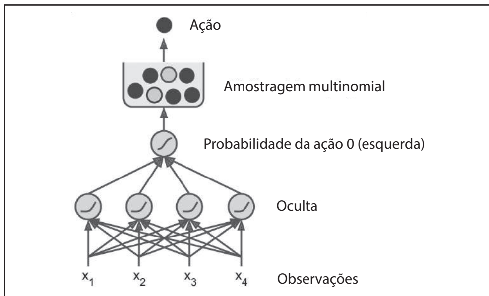
Figura 16-5. Política de Rede Neural
