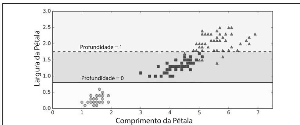
Figura 6-8. Sensibilidade aos detalhes no conjunto de treinamento
