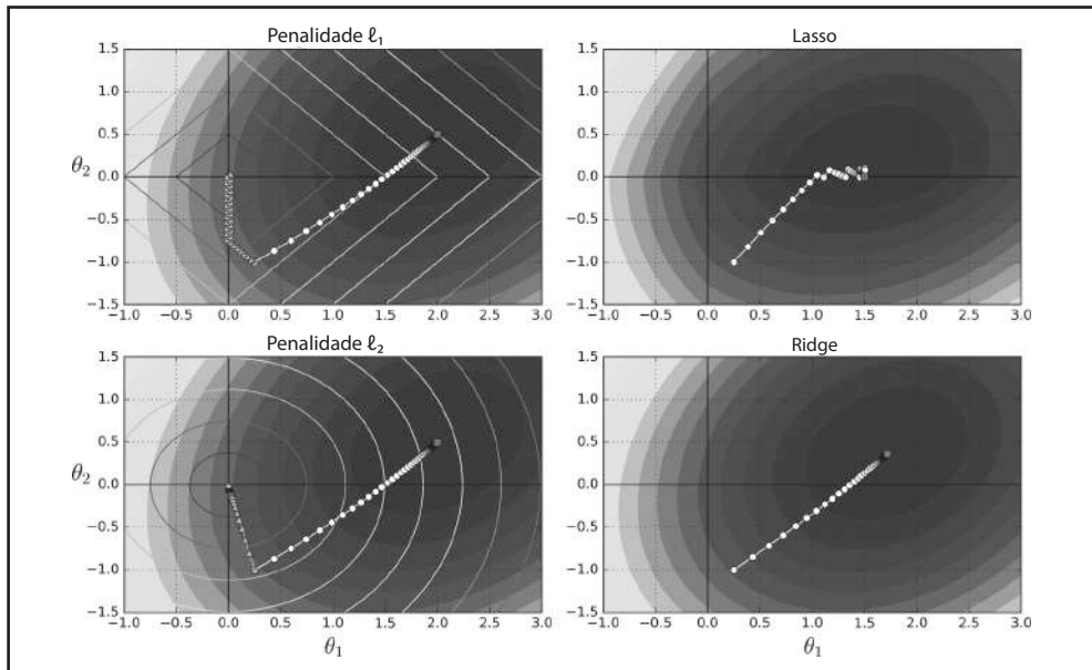
Figura 4-19. Regularização Lasso versus Ridge
