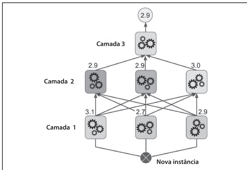
Figura 7-15. Previsões em um ensemble stacking de multicamadas
