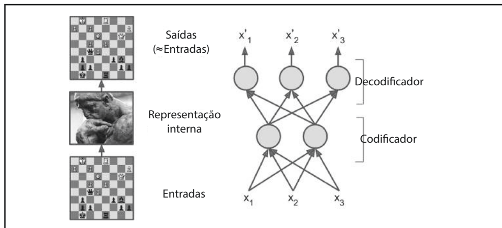
Figura 15-1. O experimento de memória do xadrez (esquerda) e um autoencoder simples (direita)
