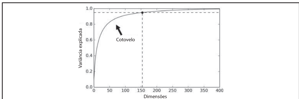
Figura 8-8. Variação explicada como uma função do número de dimensões
