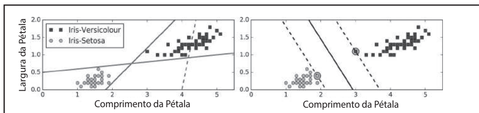
Figura 5-1. Classificação de margens largas
