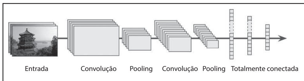
Figura 13-9. Arquitetura CNN típica
