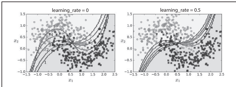
Figura 7-8. Fronteiras de decisão de previsores consecutivos
