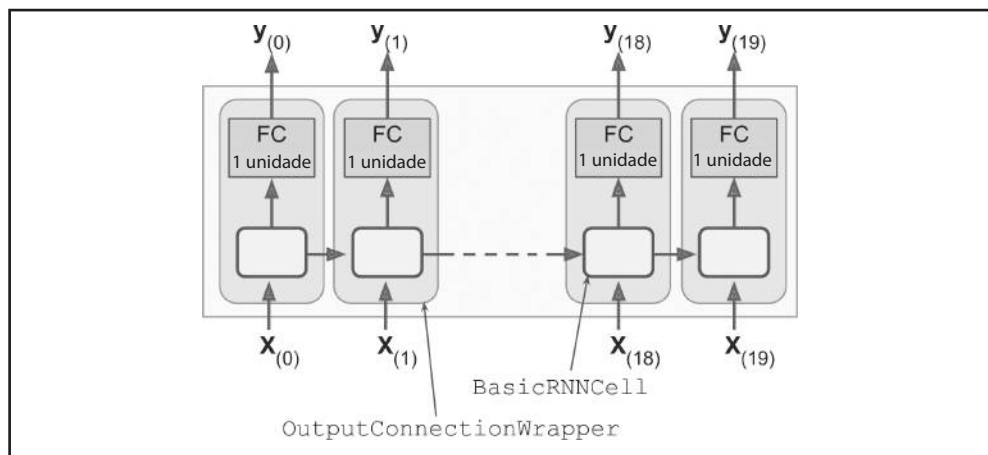
Figura 14-8. Células RNN utilizando projeções de saída
