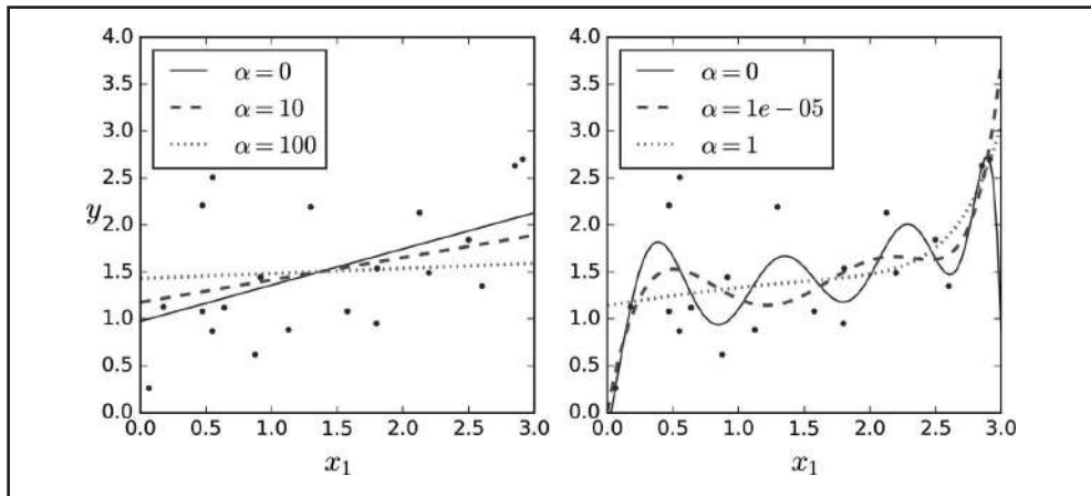
Figura 4-17. Regressão de Ridge
